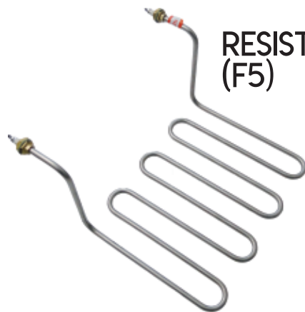
RESISTÊNCIA (F4)
